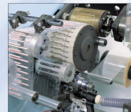
SEALING WRAPPING MECHANISM (JS-602U) 成型與切口之廢料收集 (JS-602U)
